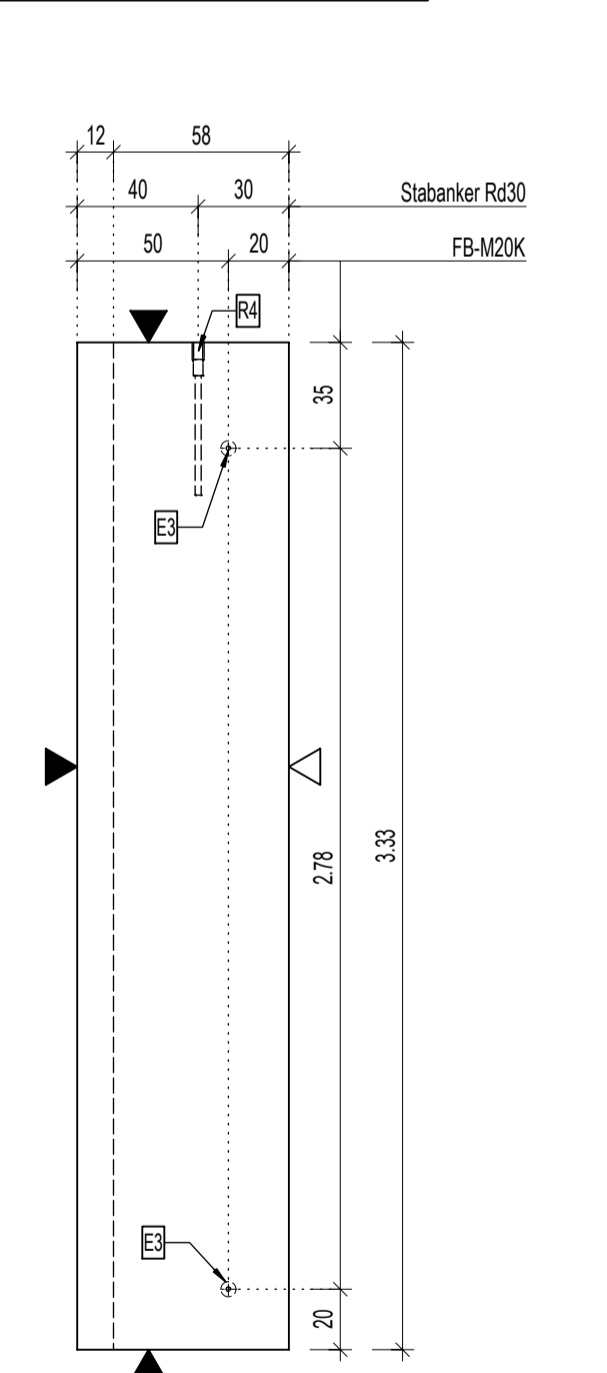
Seitenansicht von links
