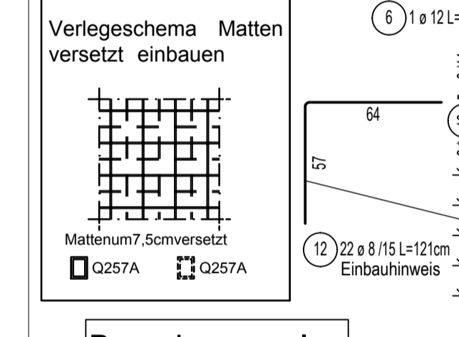
Bewehrungsplan
