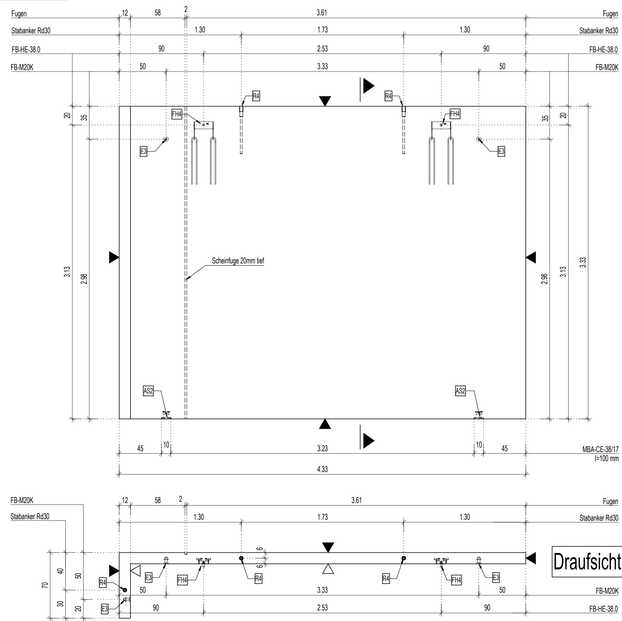
Blick in die Schalung
