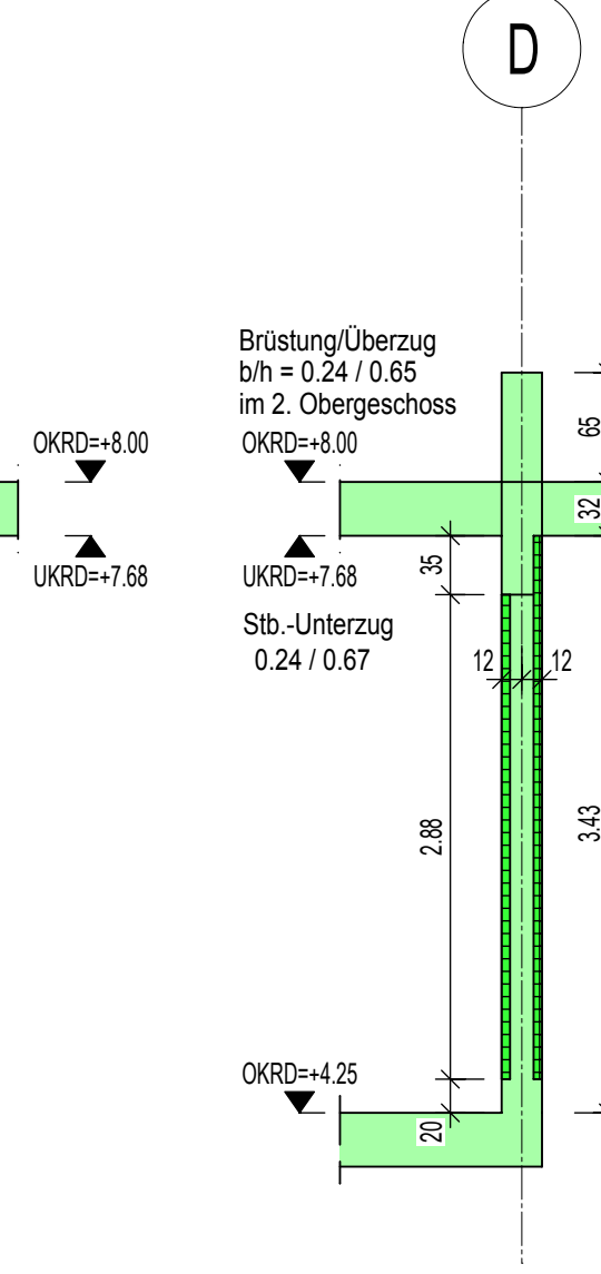
Schnitt 3.8 - 3.8 M 1:50
