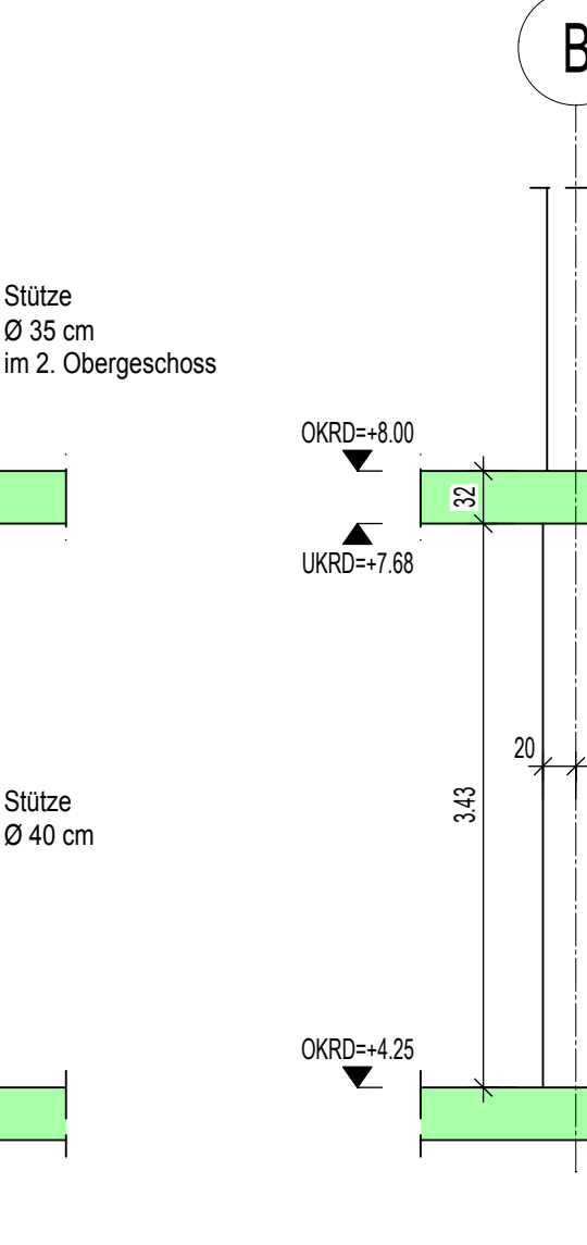
Schnitt 3.6 - 3.6 M 1:50
