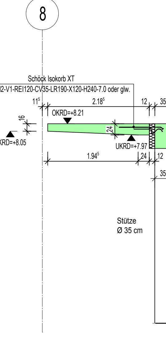
Schnitt 3.7 - 3.7 M 1:50
