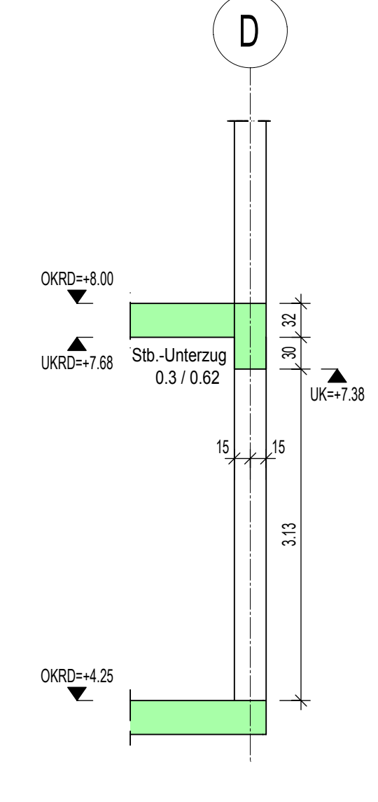
Schnitt 3.1 - 3.1 M 1:50
