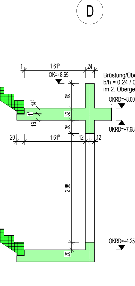
Schnitt 3.3 - 3.3 M 1:50
