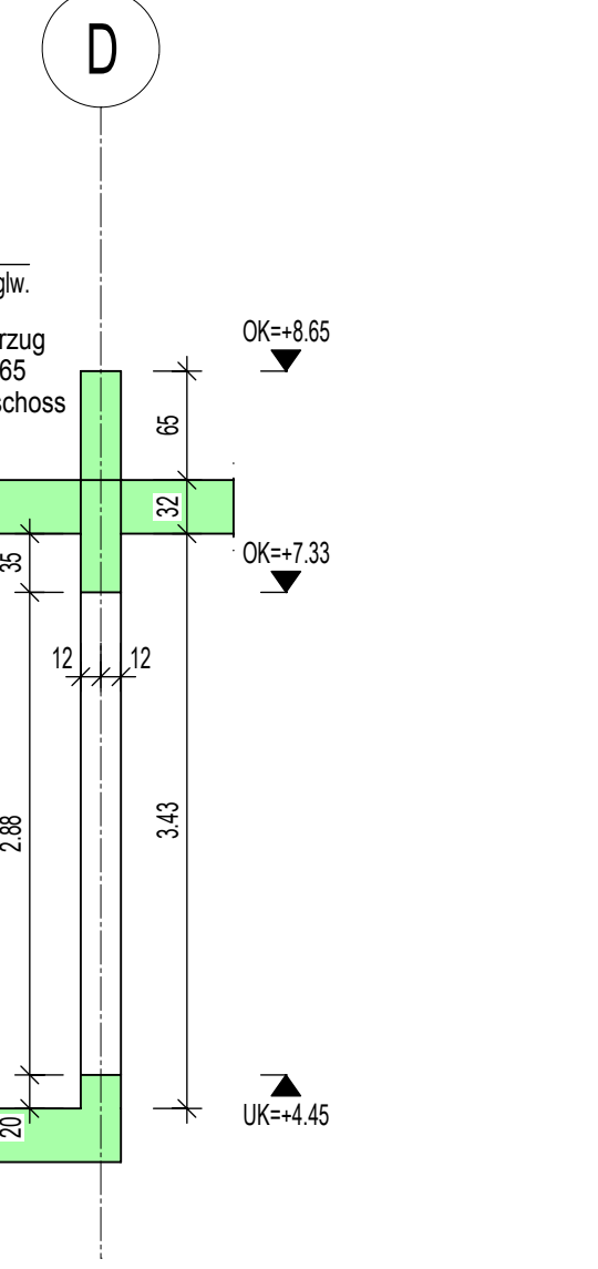
Schnitt 3.5 - 3.5 M 1:50
