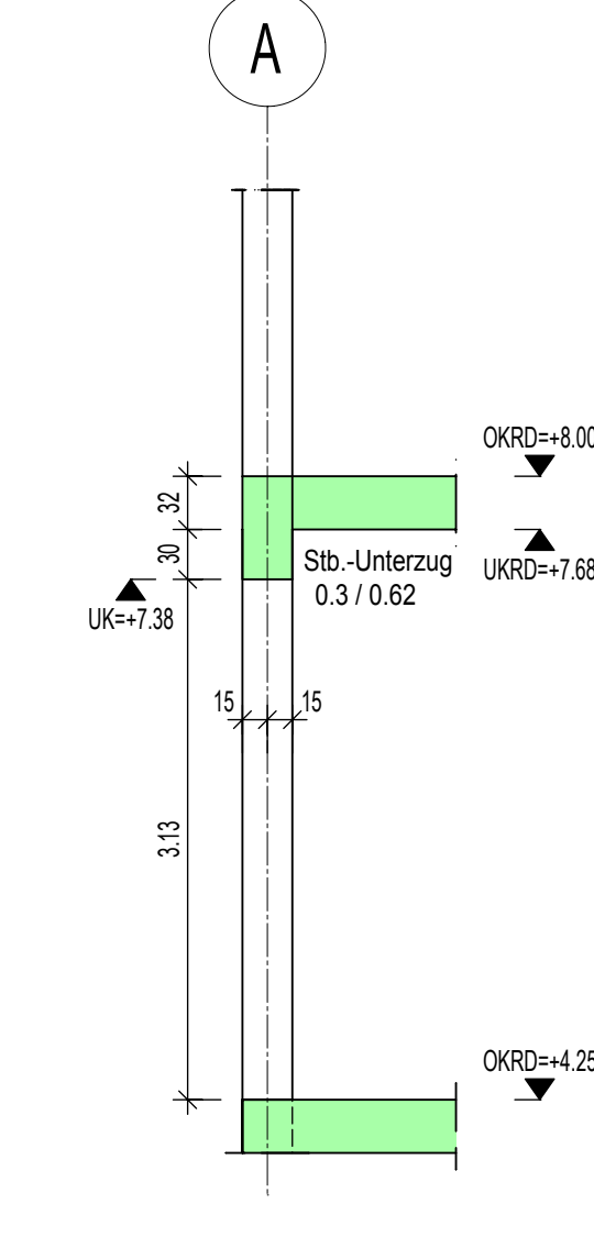
Schnitt 3.2 - 3.2 M 1:50
